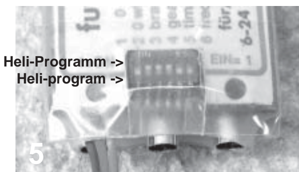
Schrumpfschlauch zurückgeklappt und mit Klebefolie fixiert Heat shrinking tubes folded back and fixed by adhesive tape
